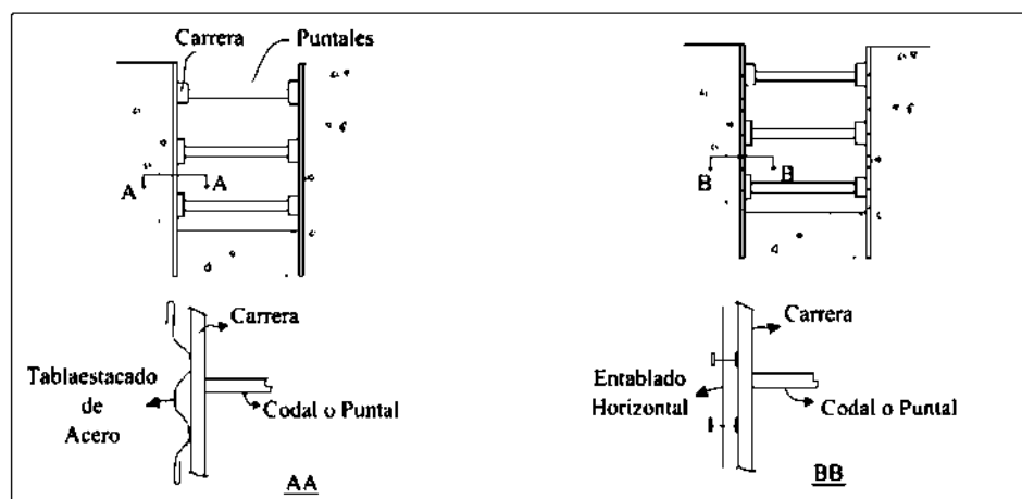
(1) Tablestacado Vertical de Acero.
