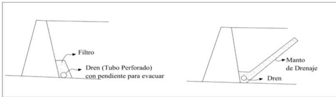
a c. Dren Lateral
