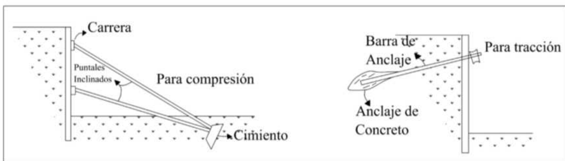
Puntales inclinados con Cimentación temporal Tierra
