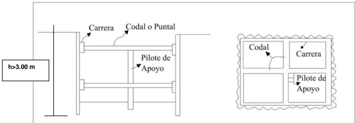
Elevación y planta de entibación cruzada
