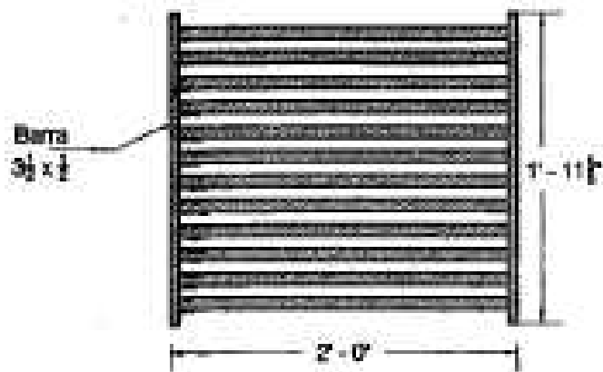
FIGURA N° 12 REJILLA CUADRADA
