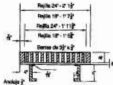
SECCION TRANSVERSAL (A través de Marco y Rejilla)
