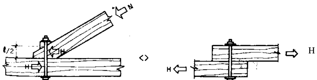
Fig. 10.3.2.7 Unión emperrada sometida a cizallamiento y fuerza axial
