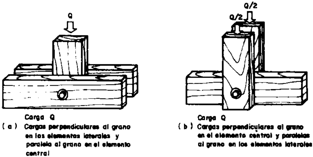
Fig. 10.3.2.2a Unión emperrada a doble cizallamiento. Cargas paralelas al grano en todos los elementos (Carga P).
