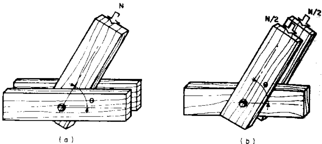
Fig. 10.3.2.3 Unión emperrada, cargas inclinadas con relación al grano
