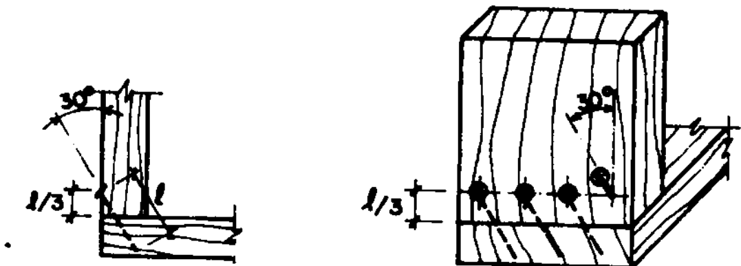
Fig. 10.2.4.1c Ubicación de clavos lanceros.
