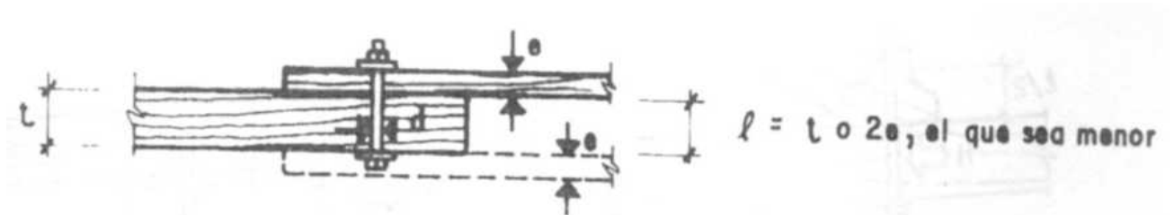
Fig. 10.3.2.5 Unión emperrada sometida a cizallamiento simple.
